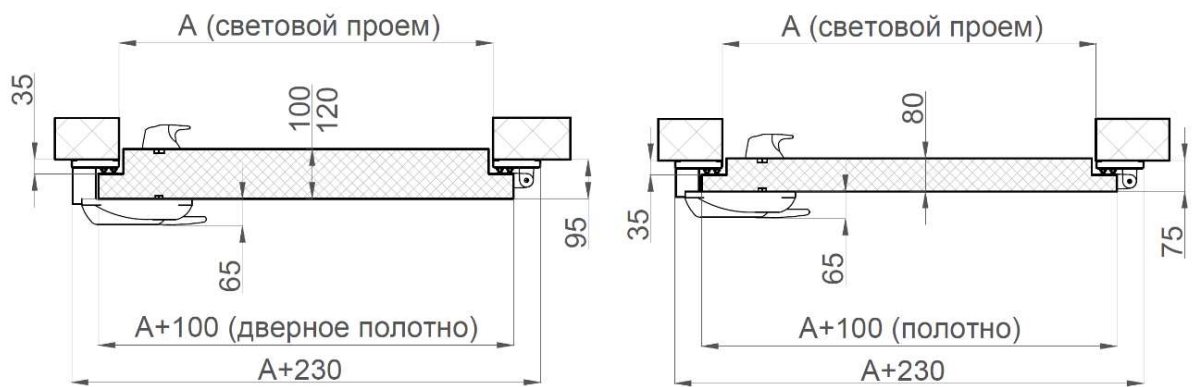
Рисунок 6. Разрез А-А. Слева – толщина полотна 100 или 120; справа толщина полотна 80 мм
