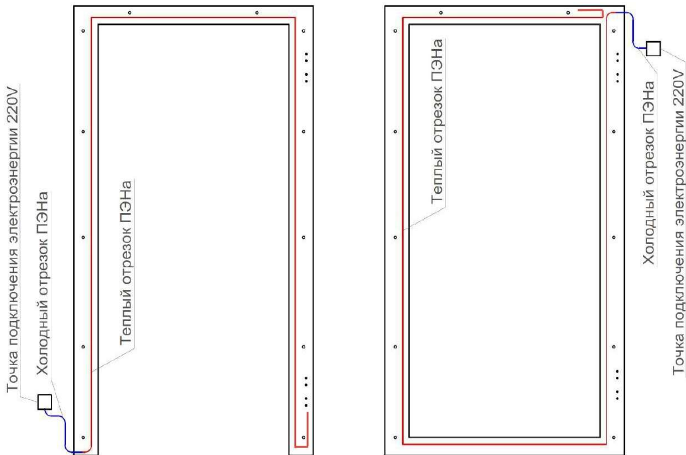
Рисунок 13. Схема расположения электронагревательного провода в накладной раме. Слева – исполнение рамы без порога; справа – с порогом
