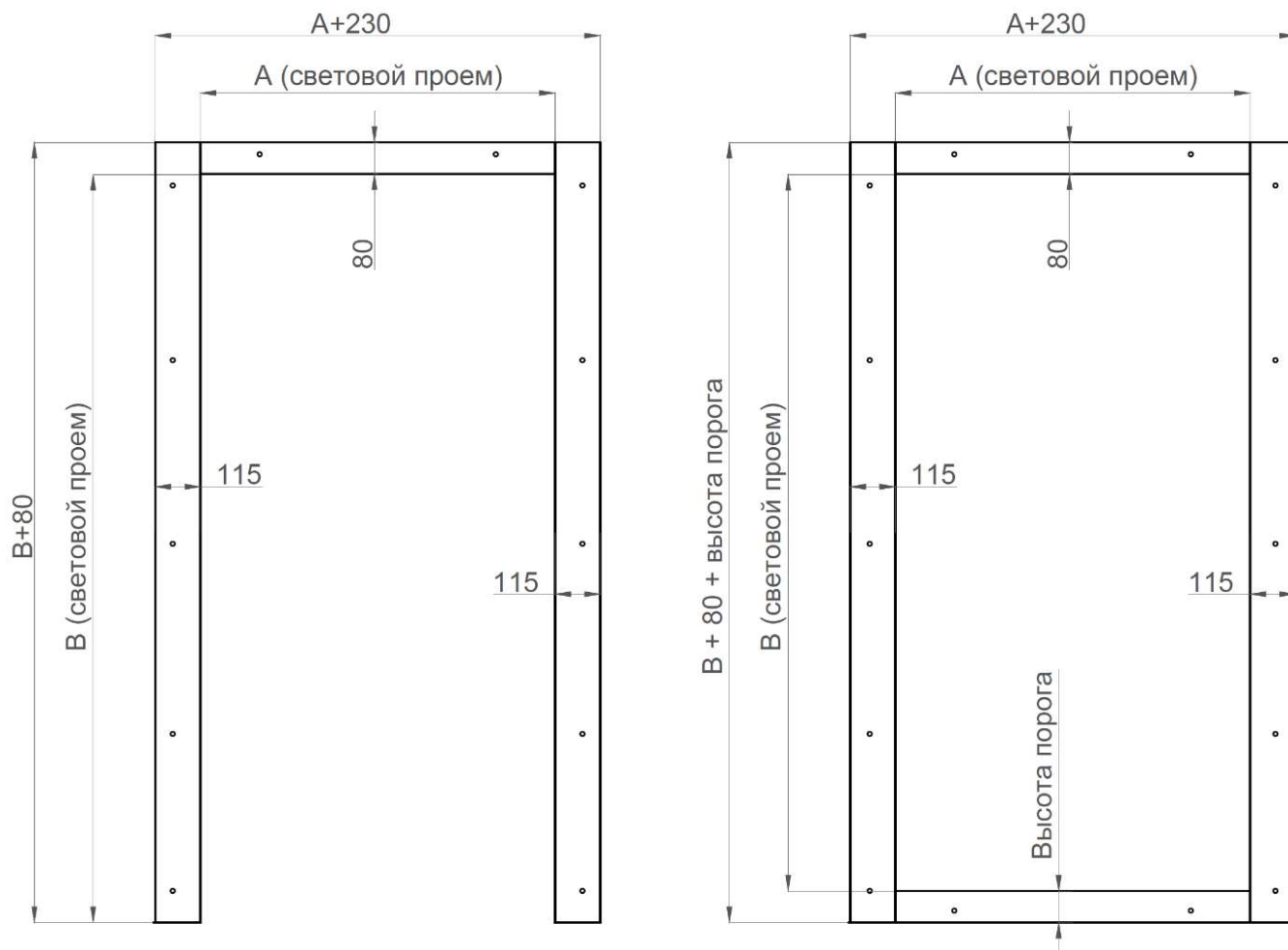
Рисунок 4. Металлическая накладная рама для РДО. Слева – без порога, справа – с порогом
