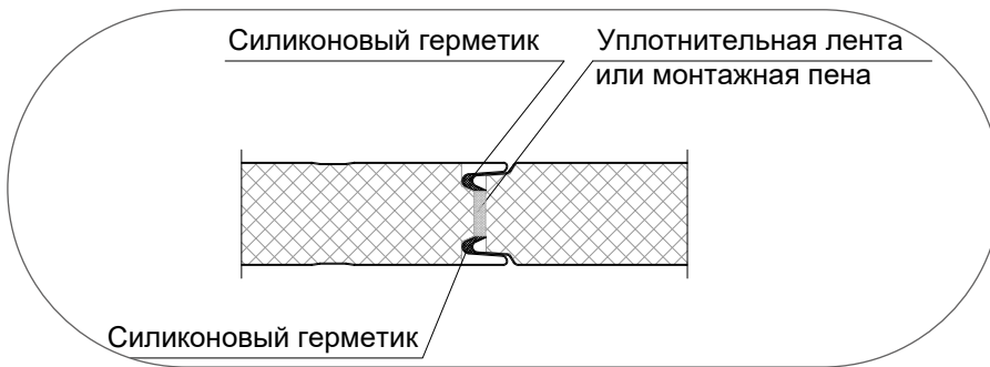
Рисунок 16. Геометрия стеновой сэндвич-панели с замковым соединением Z-Lock (ПСТ Z)
