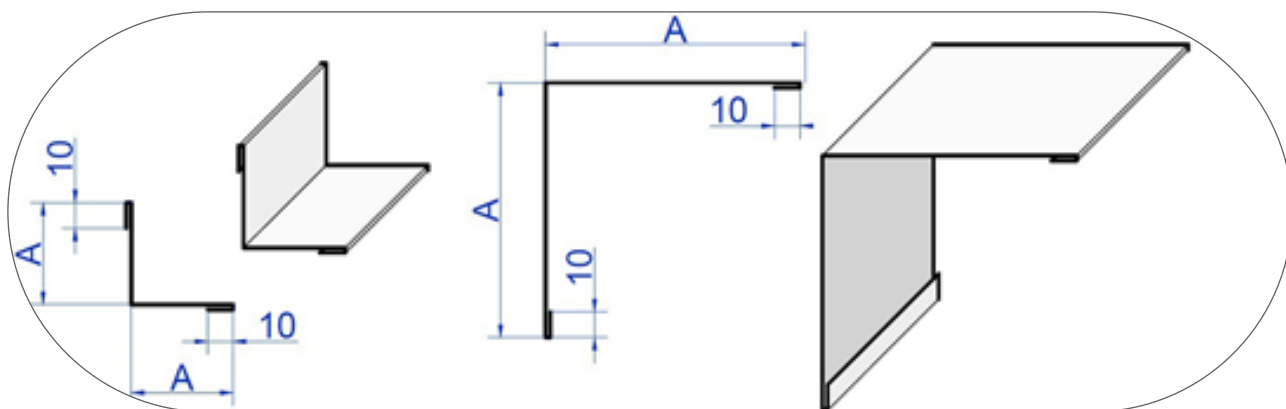
Рисунок 39. Равносторонние уголки (плоские)
