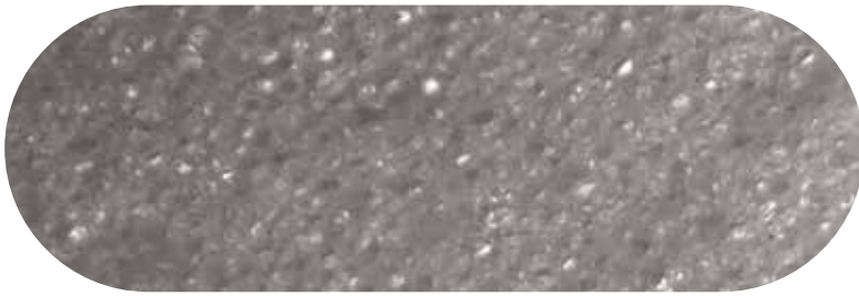
Рисунок 2. Ячеистая структура ППУ с 20-кратным увеличением. Шкала деления 0,5 мм
