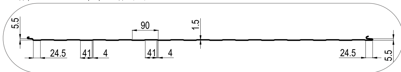
Стандартная накатка «ПроФХолода» (РН)
