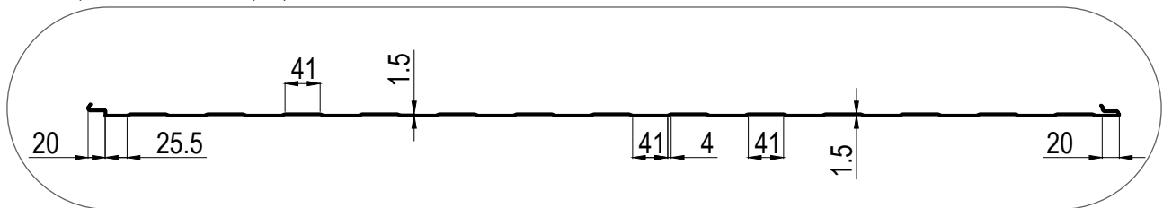
Рисунок 14. Виды профилировки внутренней стороны сэндвич-панелей ПСТ Стандартная накатка «ПрофХолода» (РН)
