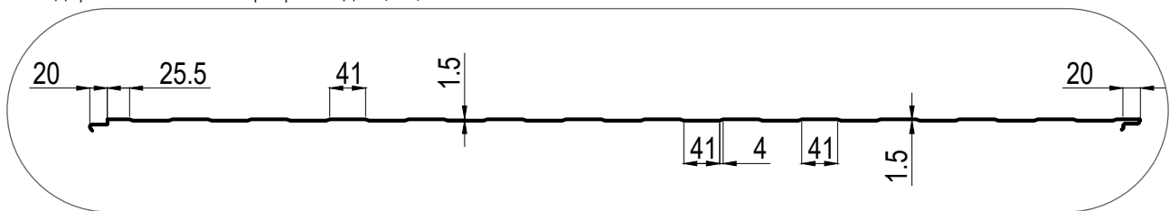
Без накатки «ПрофХолода» (Гл)
