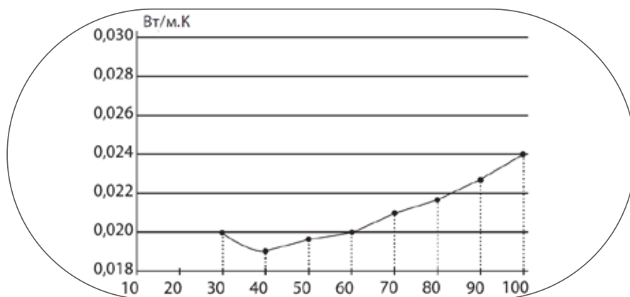
Рисунок 5. Зависимость теплопроводности от плотности ППУ
