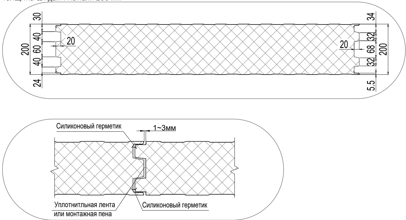
Рисунок 13. Стык стеновых панелей со стандартным замковым соединением Стандартная накатка «ПрофХолода» (РН)
