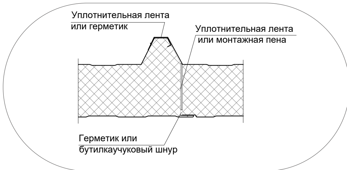
Рисунок 25. Стык кровельных панелей со стандартным замковым соединением
