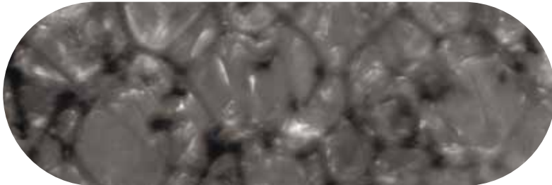
Рисунок 3. Ячеистая структура ППУ с 300-кратным увеличением. Шкала деления 0,5 мм
