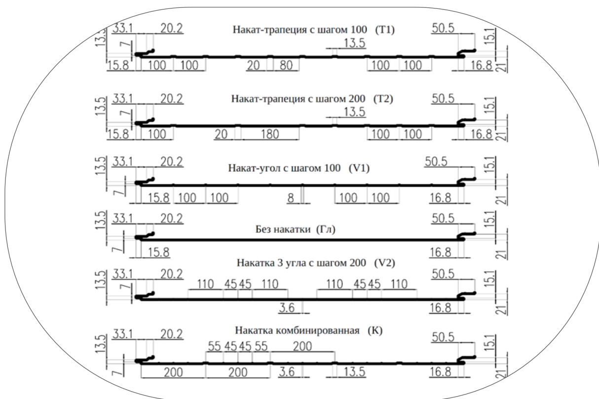
Рисунок 22. Виды профилировки внутренней стороны сэндвич-панелей ПСТ SF
