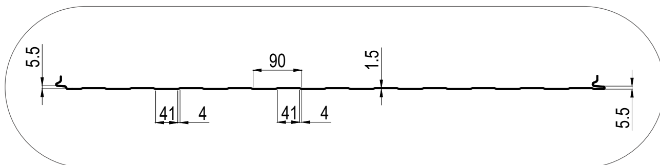
Накат-трапеция с шагом 100 (Т1)
