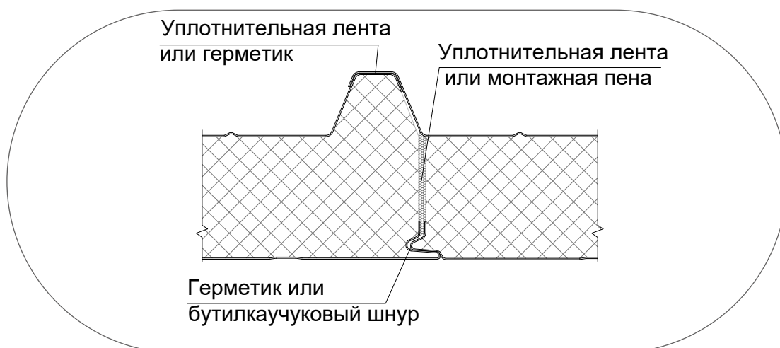
Рисунок 29. Стык кровельных сэндвич-панелей с замковым соединением Z-Lock
