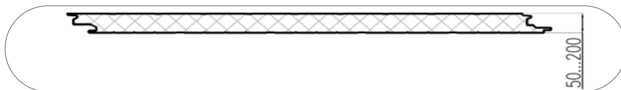
Рисунок 19. Виды профилировки внутренней стороны сэндвич-панелей ПСТ Z
