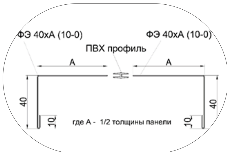
Рисунок 36-1. Профиль для обрамления светового проема в панели
