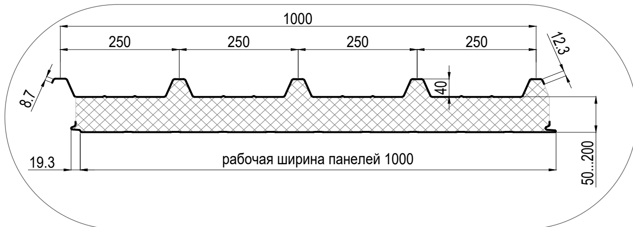
Рисунок 28. Геометрия кровельной сэндвич-панели с замковым соединением типа Z-Lock (ПКТ Z)
