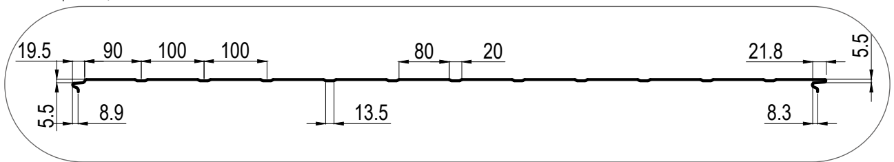
Рисунок 17. Стык стеновых панелей с замковым соединением Z-Lock Накат-трапеция с шагом 100 (Т1)
