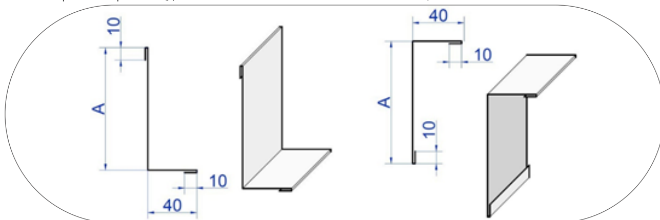
Рисунок 41. Уголки неравносторонние (для стыков потолочных и стеновых панелей)
