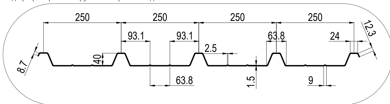
Рисунок 31. Вид профилировки наружной стороны сэндвич-панелей ПКТ Z
