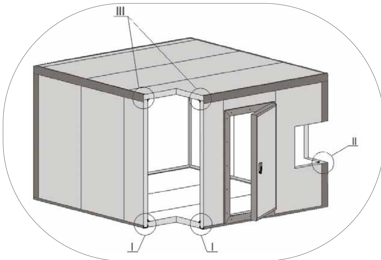
Рисунок 34. Основные узлы стыковки сэндвич-панелей для сборки холодильных камер (начало)
