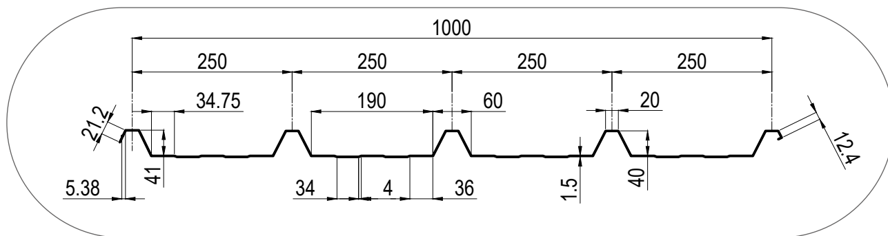
Рисунок 27. Вид профилировки наружной стороны сэндвич-панелей ПКТ
