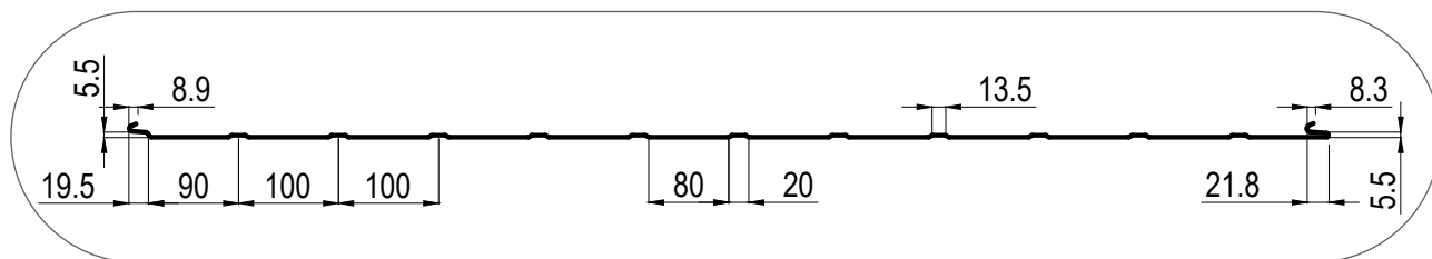
Накат-трапеция с шагом 200 (Т2)
